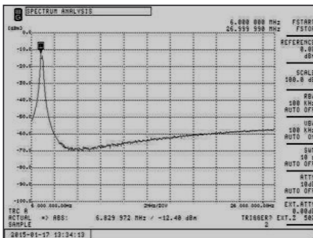
Curva di risposta a 6.8Mc; Banda 7....29 BW stretta; Attenuaz. ca 12.5dB; Selettività molto alta , a 100Kc - 14dB
