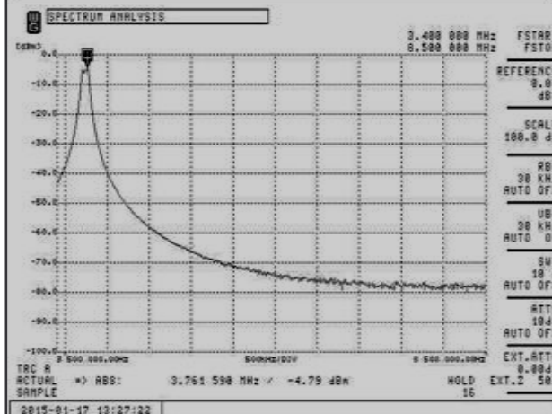
Curva di risposta a 3.7 Mc; Banda 3.6..... 7.1 BW stretta; Attenuaz. ca 4.8dB
