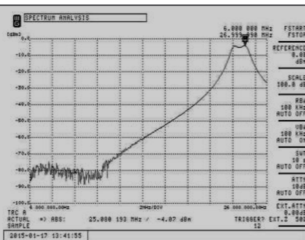
Curva di risposta a 25Mc; Banda 7.....29 BW larga; Attenuaz. ca 4dB
