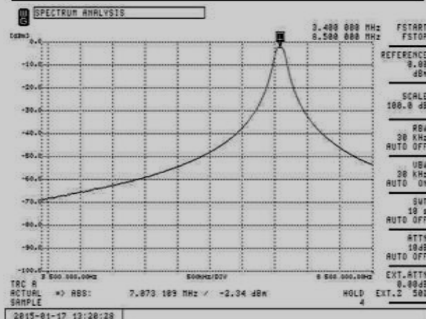
Curva di risposta a 7.1 Mc; Banda 3.6..... 7.1 BW stretta; Attenuaz.2.3dB; a 100Kc -12dB
